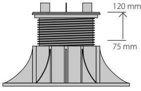
Supporto a testa autolivellante
