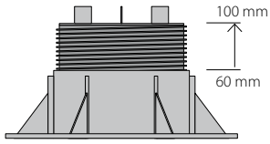
Supporto a testa fissa
